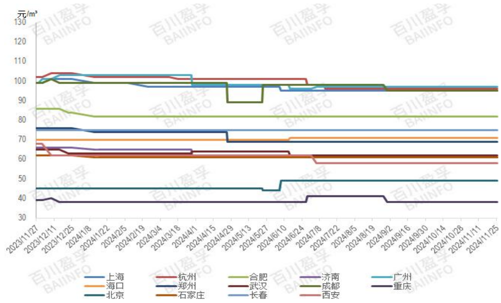
图：本月全国重点城市机制砂价格走势
