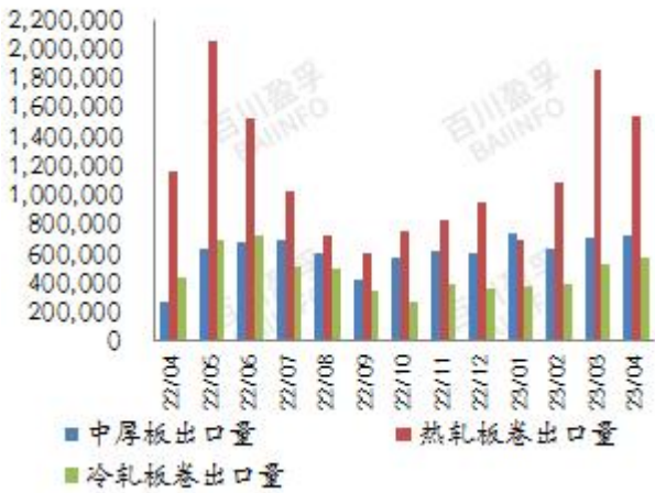
图 61：国内板材出口量走势（吨）
