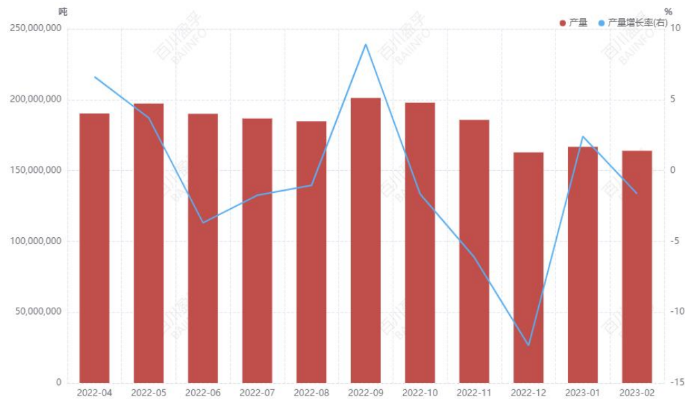
图：2022 年 4 月-2023 年 2 月全国水泥总产量对比图
