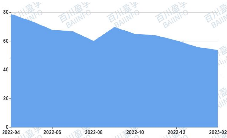
图： 2022 年 4 月-2023 年 2 月全国水泥行业开工率走势图
