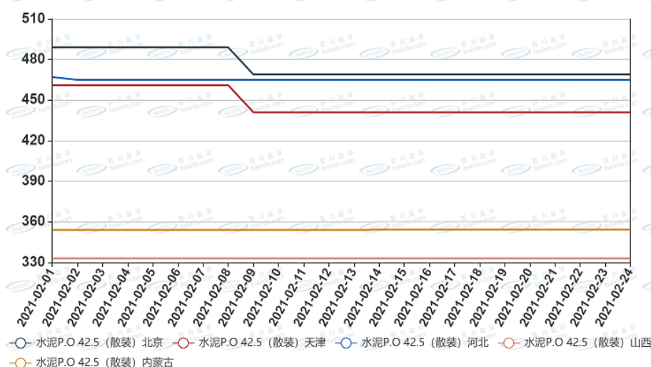
图：本月华北地区水泥价格走势
