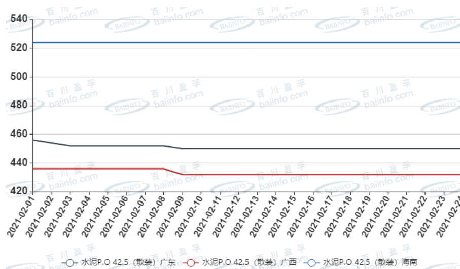
图：本月华南地区水泥价格走势
