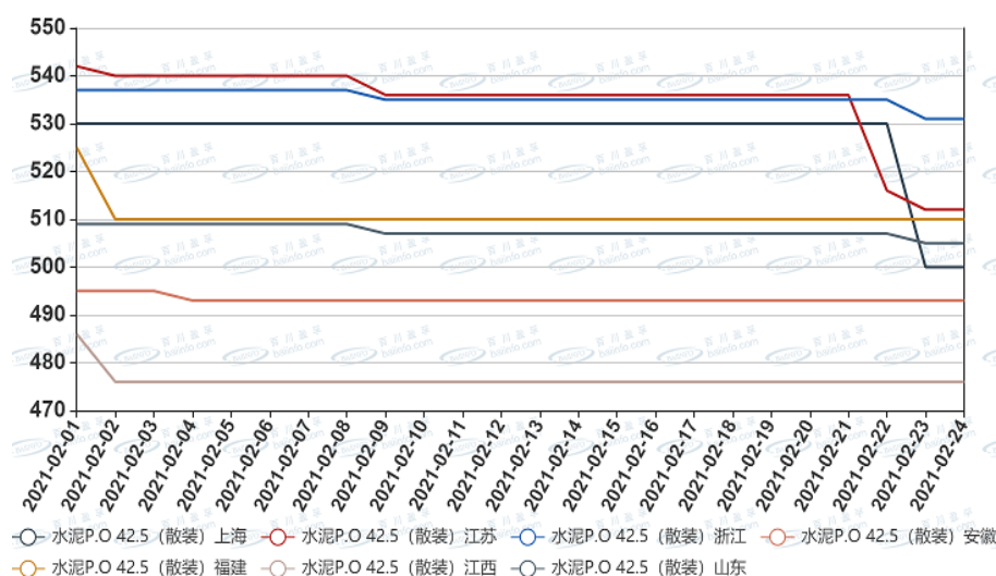
图：本月华东地区水泥价格走势
