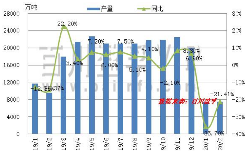
2019年1月-2020年2月水泥产量走势图
