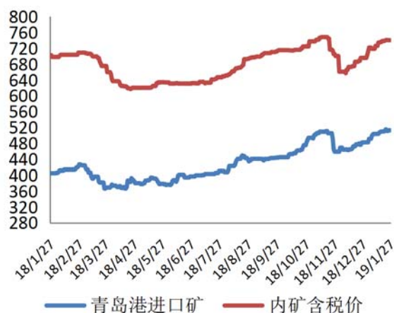
图 12: 国产矿、进口矿价格走势 (元/吨)
