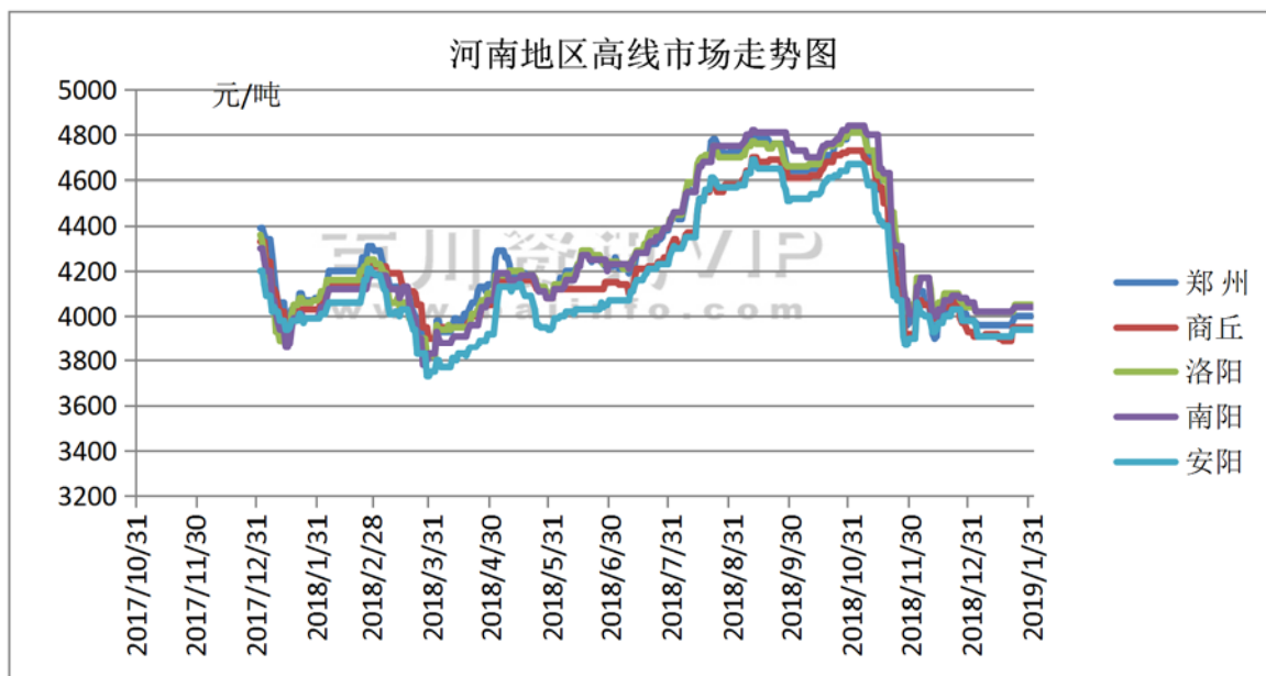
河南地区高线市场走势图
