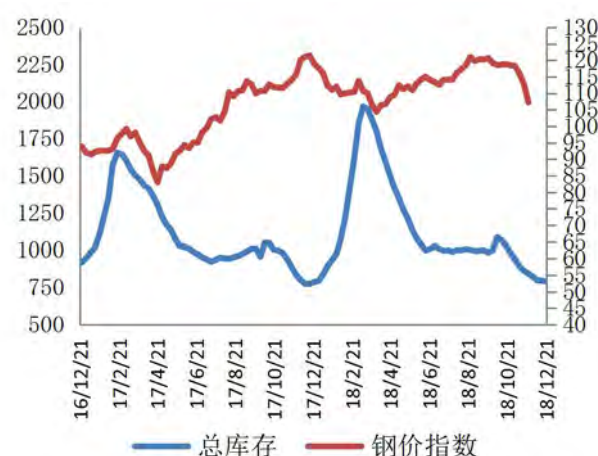
图 44：全国板材总库存走势（万吨）
